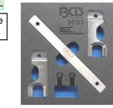
MB6 Balansas instel gereedschap. Outils de réglage d'arbre d'équilibrage Mercedes OM651 (gebruiken met / utiliser avec MB3. OEM 651 589 02 63 00
