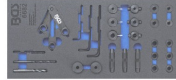
BGS6682 Cilinderkop-boormal gereedschapset voor gebroken of afgescheurde bouten. Op uit & inlaatspruitstukken, cilinderkoppen, versnellingsbakken, differentiëlen, motoren, behuizingen ... Extracteur de goujons de culasse cassés ou arrachés. M8 et M10 Pour collecteurs, des ponts d'admission, culasses, différentiels, etc. Moteurs, carters...
