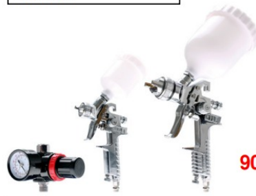
BGS3381 Verfpistolen HVLP Pistolets de peinture 125ml / 0,8mm / 600ml - 1,3mm
