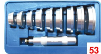
BGS1522 Dichtringen en lagers plaatser Outil pour placer bourrages et roulements 40-44-50-59-63-65-72-76-81 mm
