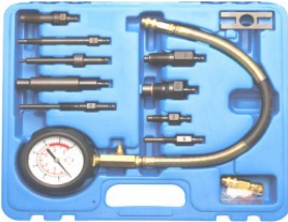
BGS8008 Compressiemeter diesel Compressiomètre 122 €
