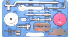
FIAT6 2,2 JTD 4HV - 2,3 JTD F1AE0481D 120PS- 2,3 JTD F1AE0481D 127PS- 3,0 JTD - PSA Puma 22DT 4HV - F30DT
